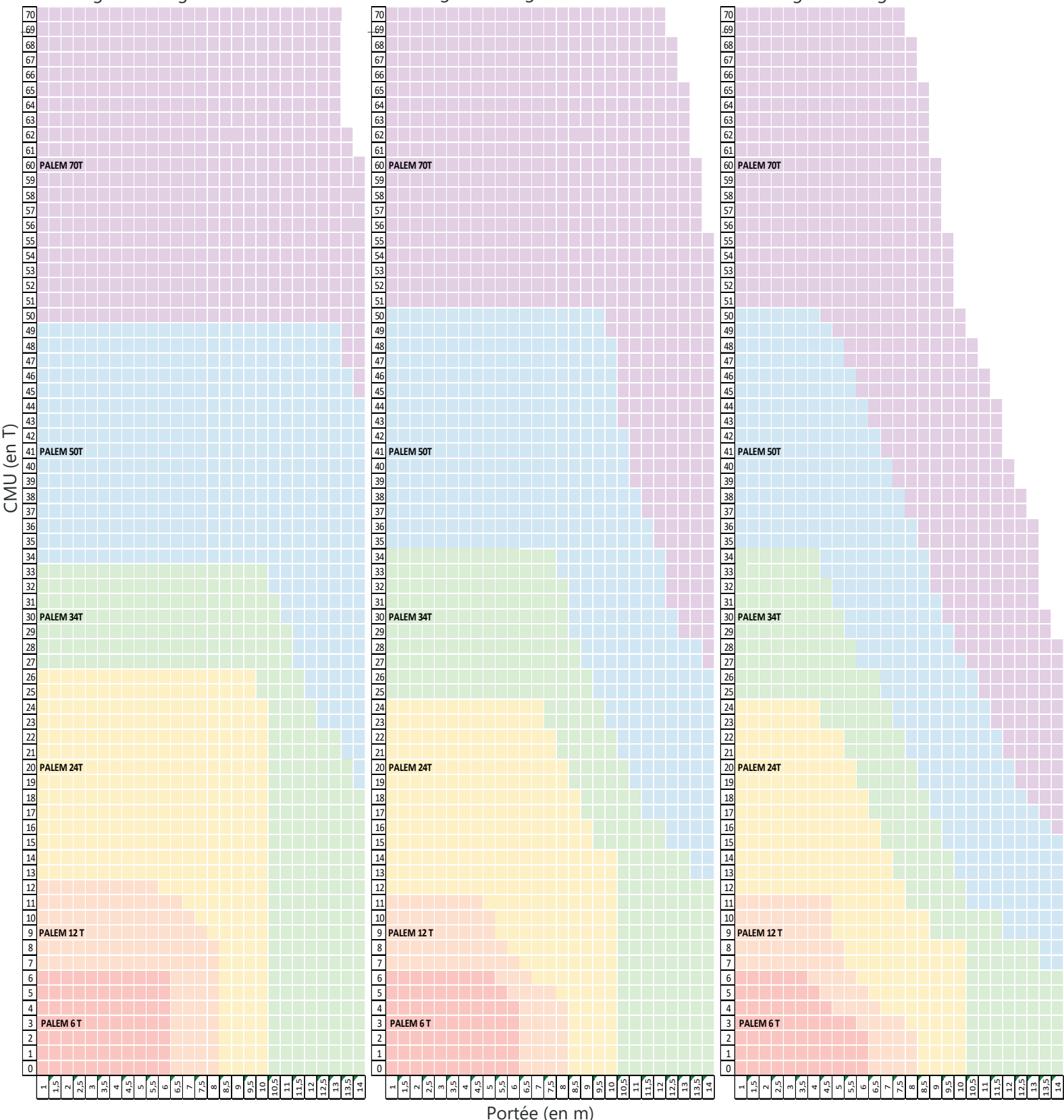
Charge avec angle de tête 40°
